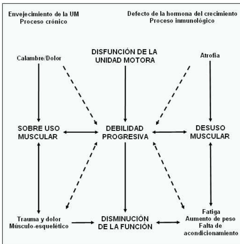
Figura 4 - Modelo esquemático que demuestra la interacción de los posibles factores etiológicos del SPP. Fuente: Halstead (1995), modificado.
